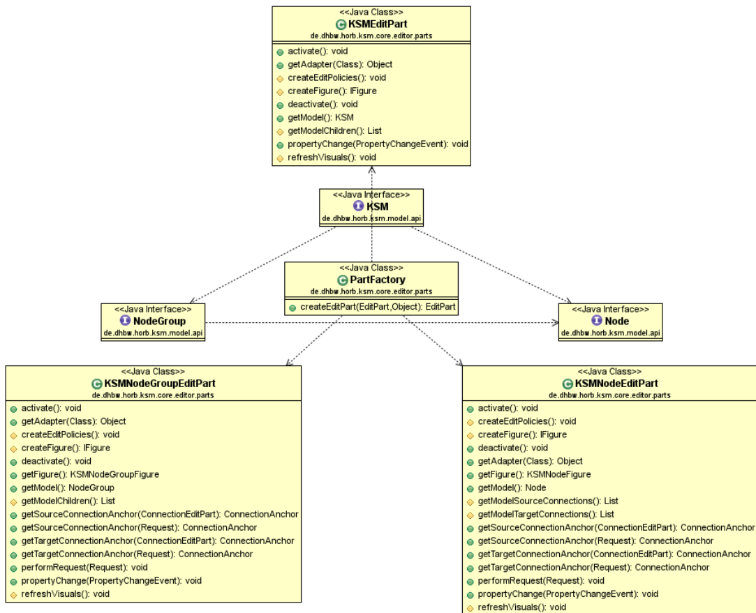
Abbildung 3.1: Model und View von KSM/NodeGroup/Node
