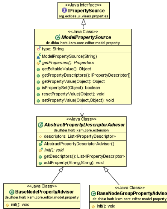
Abbildung 3.5: Klassen des Extension Point für Property Deskriptoren
