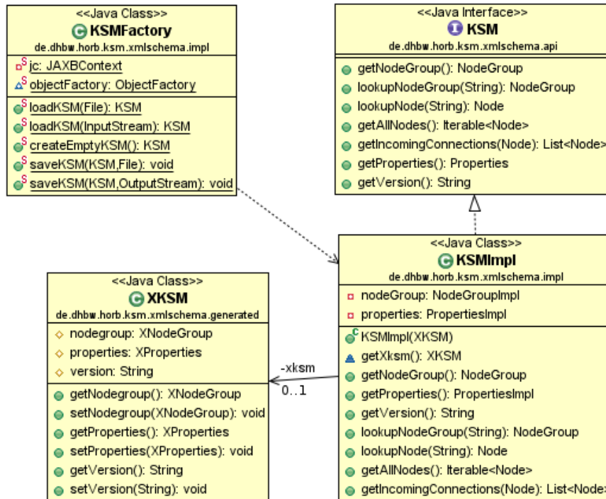
Abbildung 2.2: Klassendiagramm XML-Datenmodell Bibliothek, Ausschnitt KSM Model-Klasse
